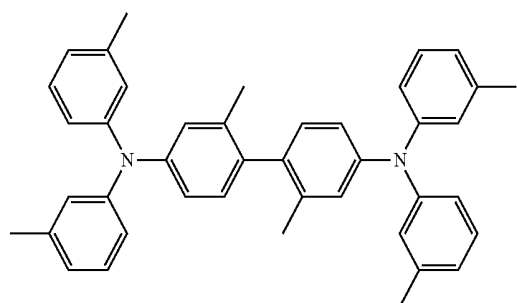
HMTPD
