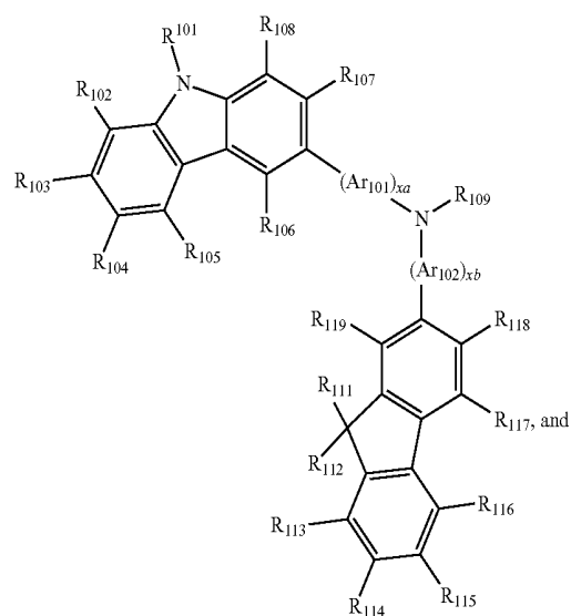
HMTPD
